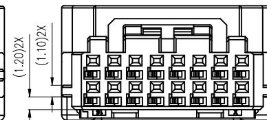
KEY-3 (16P)
