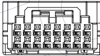
KEY-2 (16P)
