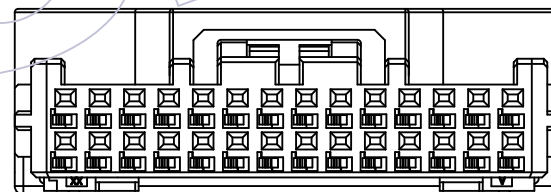
KEY-2 (28P)
