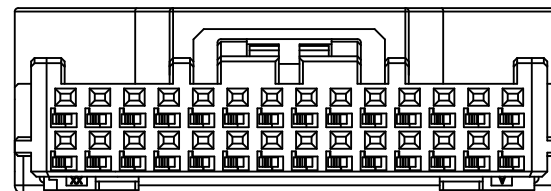
KEY-3 (28P)
