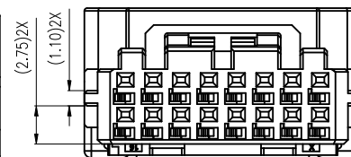
KEY-2 (16P)
