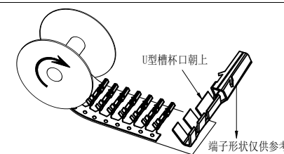
端子电镀后绕盘方向示意图
